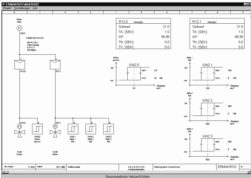
Raumregelkreis mit ER3200: Heizen / Kühlen, 3-stufige Lüfteransteuerung
